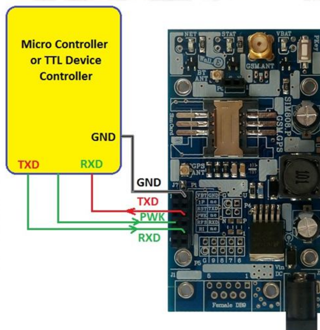
شکل 9: اتصال برد توسعه ABg184P-C به میکروکنترلر
