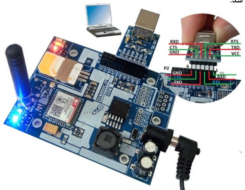
شکل 2: اتصال برد توسعه ABg144N-C به رایانه توسط مبدل یو اس بی
