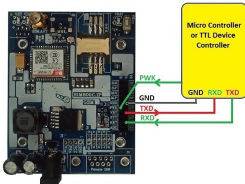
شکل 5: اتصال برد توسعه ABg144N-C به میکروکنترلر
