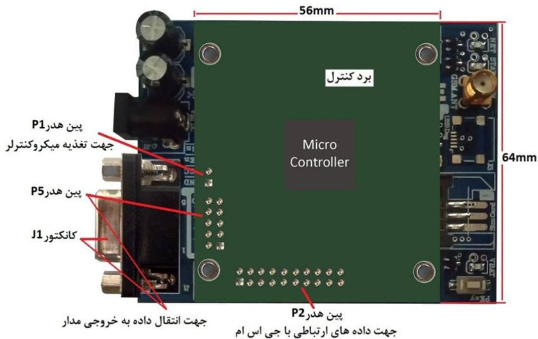
شکل 6: طراحی و نصب برد کنترل
